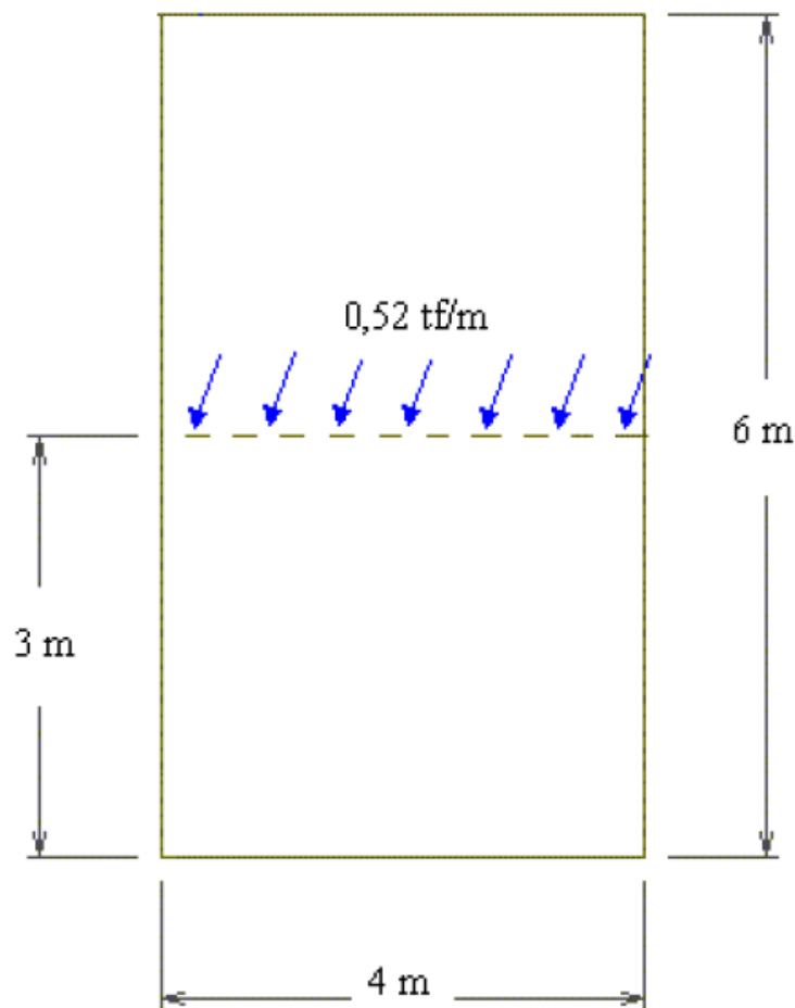
Figura 1 – Esquema da laje.
